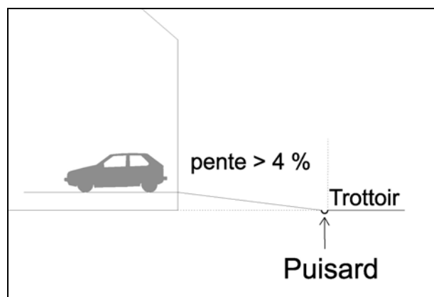
Chemin d'accès avec puisard
